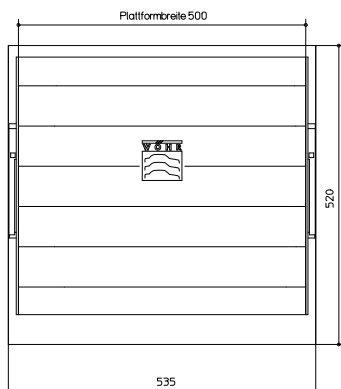
Wöhr Parklift 411 2,6 - D 500
