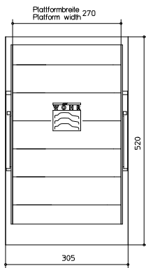
Wöhr Parklift 411 2,6 - E 270
